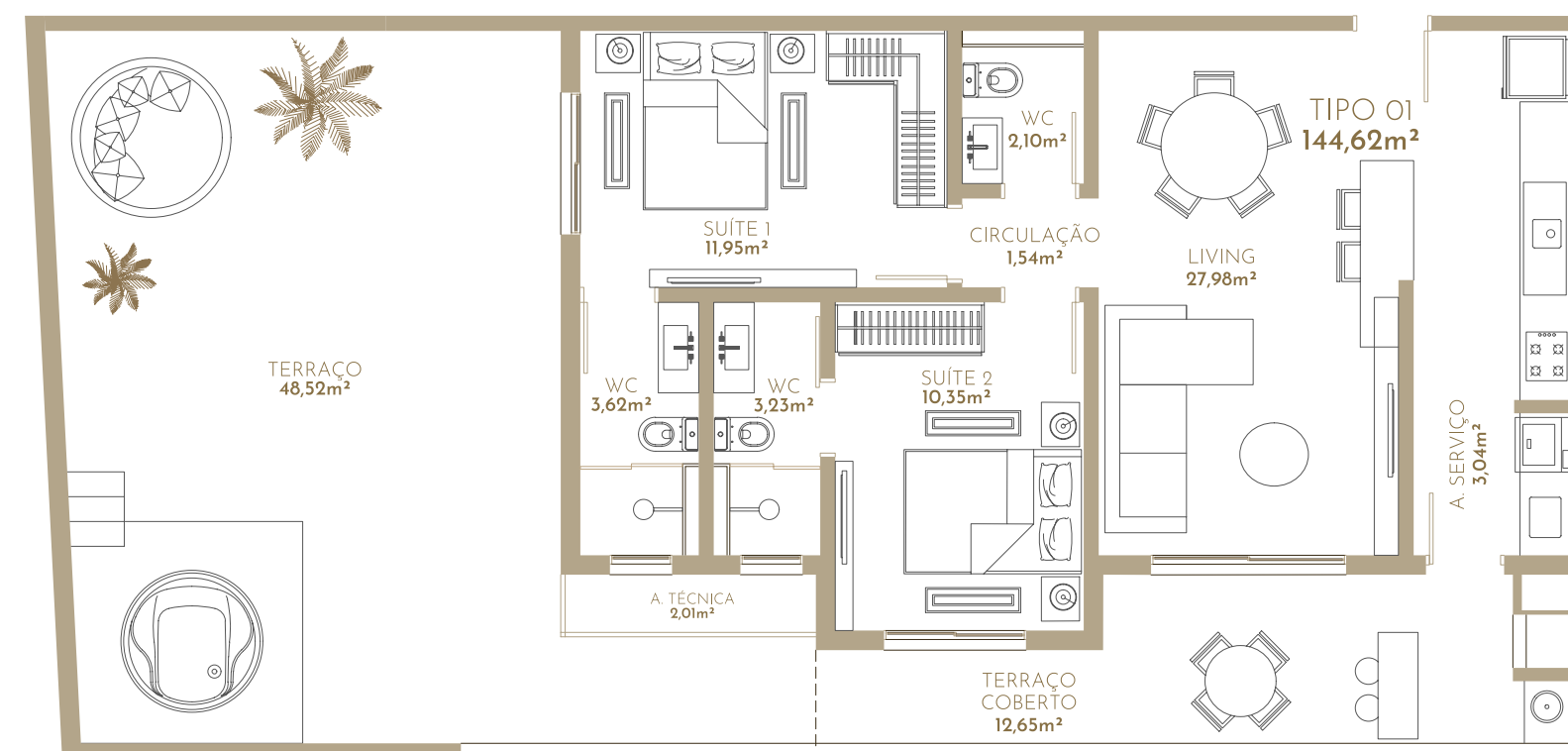
TIPO 01 144,62m 2
