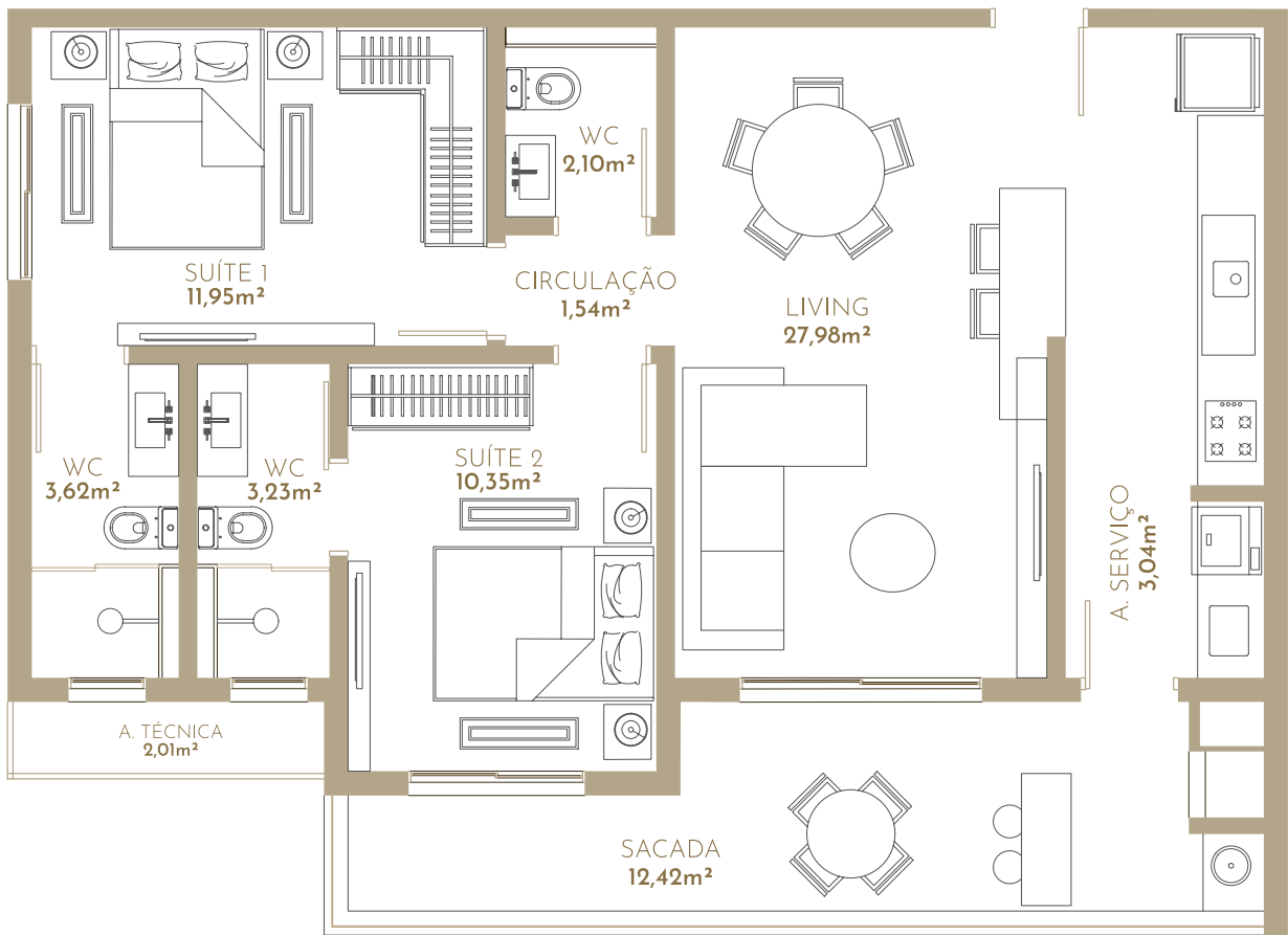
TIPO 01 92,02m²
