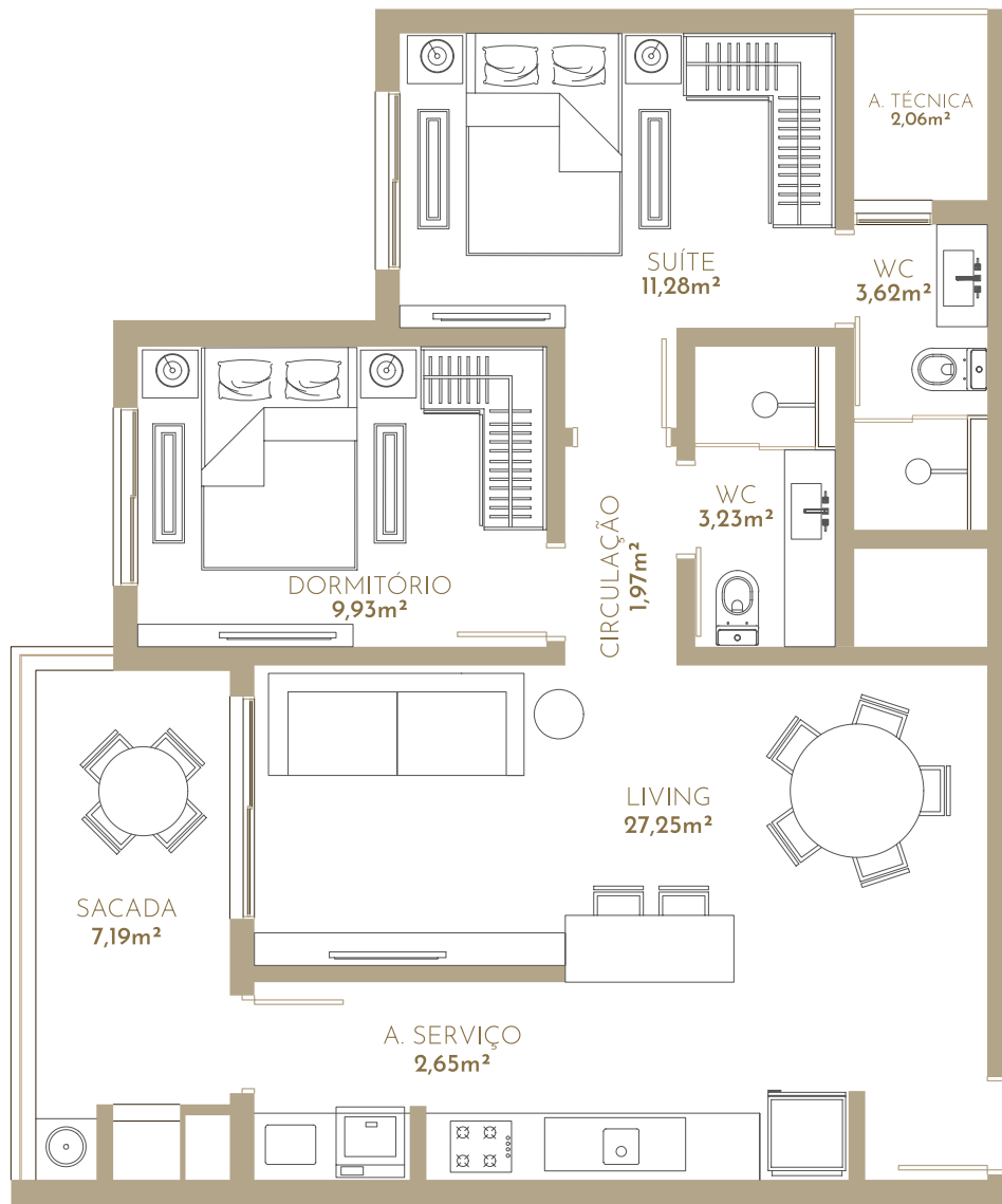
TIPO 03 81,98m²
